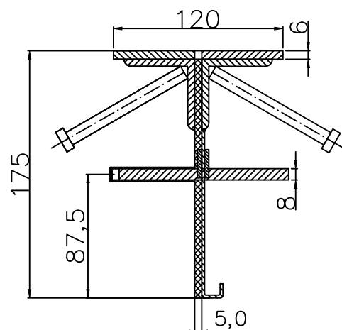
CONECTO SINUS 06NC115-5D-T8 h=175 SECTION
