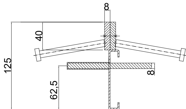
CONECTO DOWEL 08NA40-5D-T8 h=125 Section Scale 2:1
