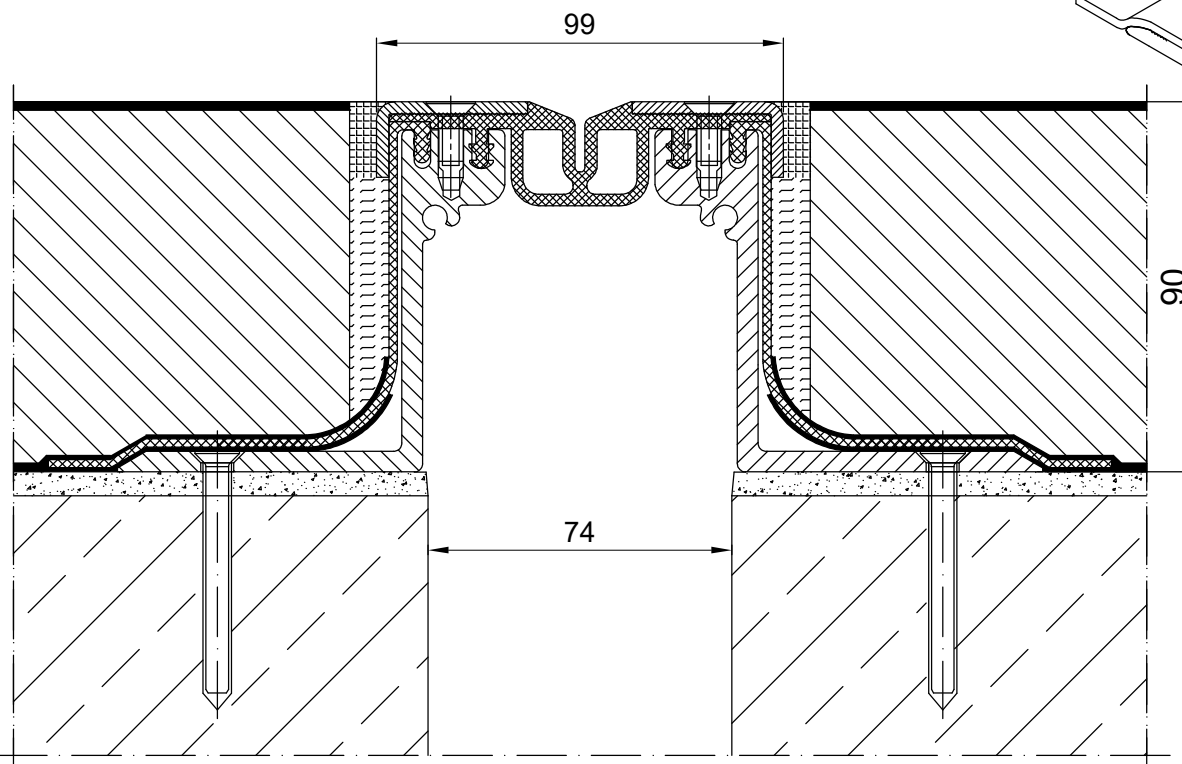
CONECTO GA 50.20.90 L Przekrój
