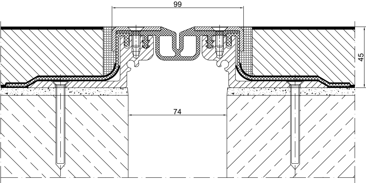
CONECTO GA 50.20.45 L SECTION
