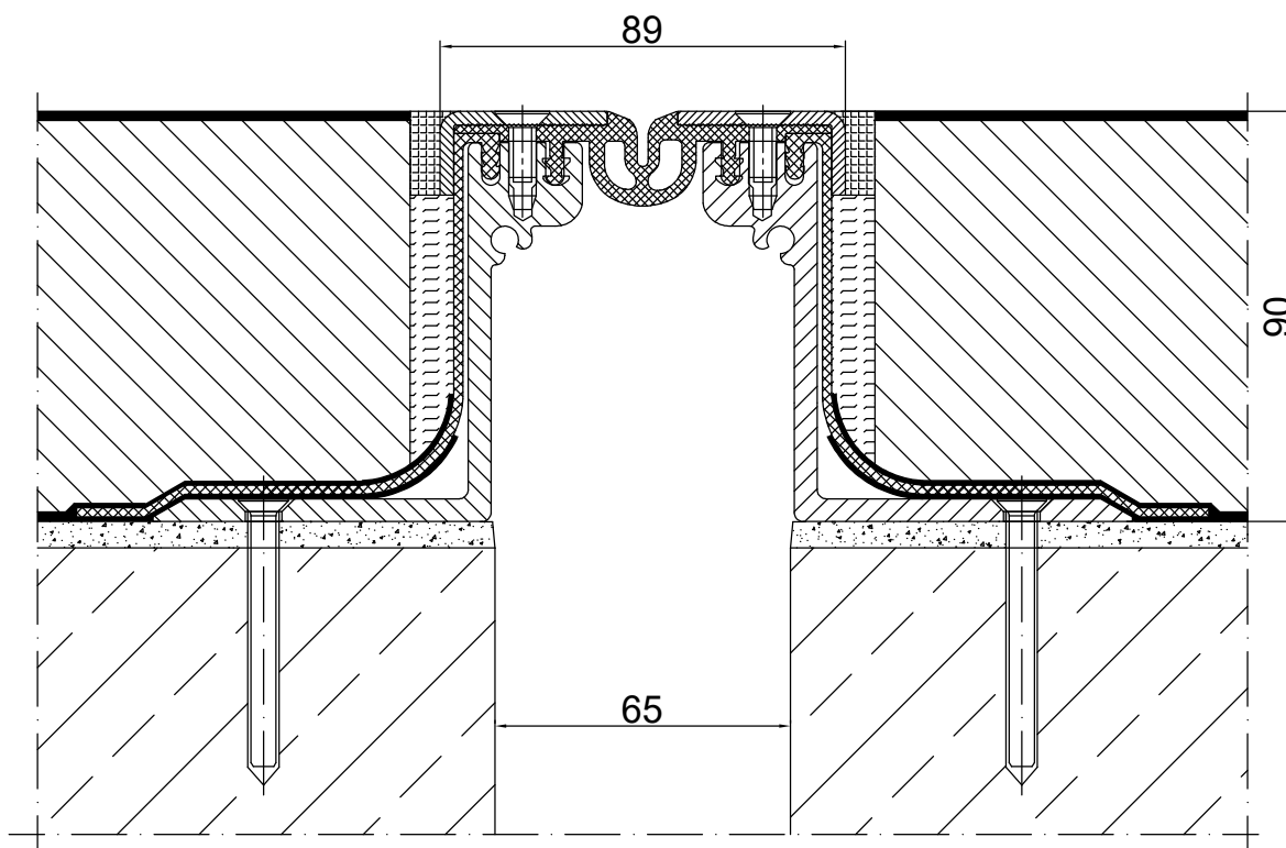
CONECTO GA 43.10.90 L SECTION
