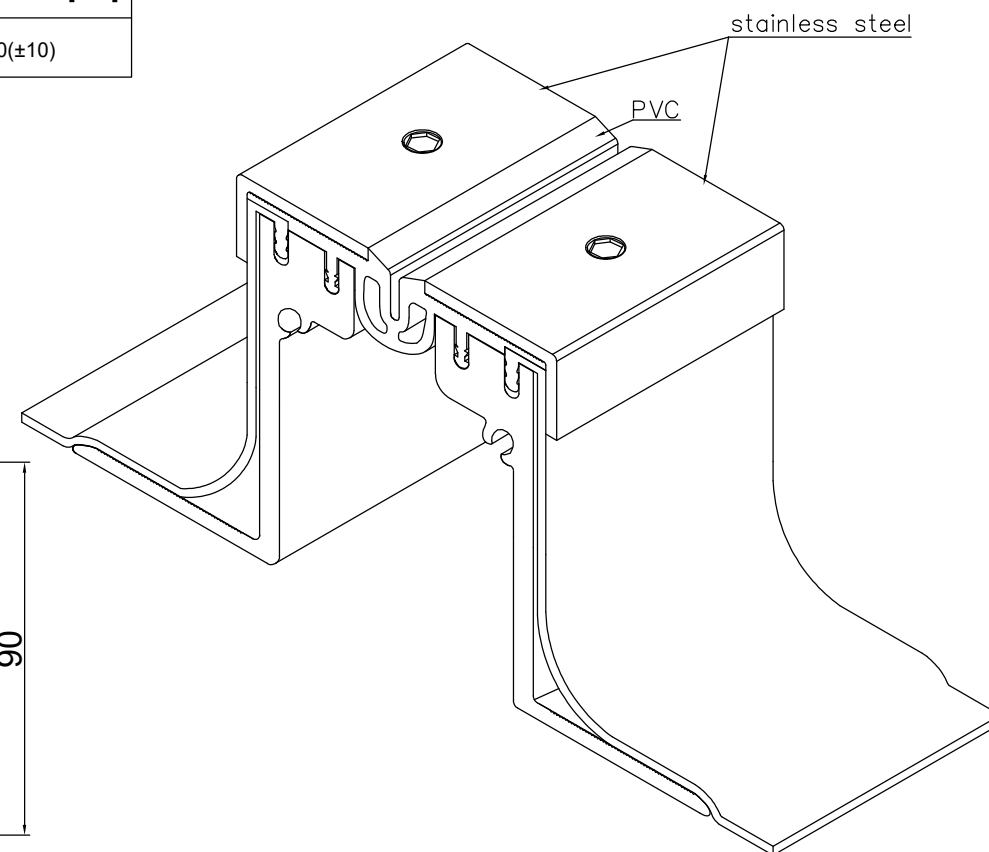
CONECTO GA 43.10.90 L VIEW
