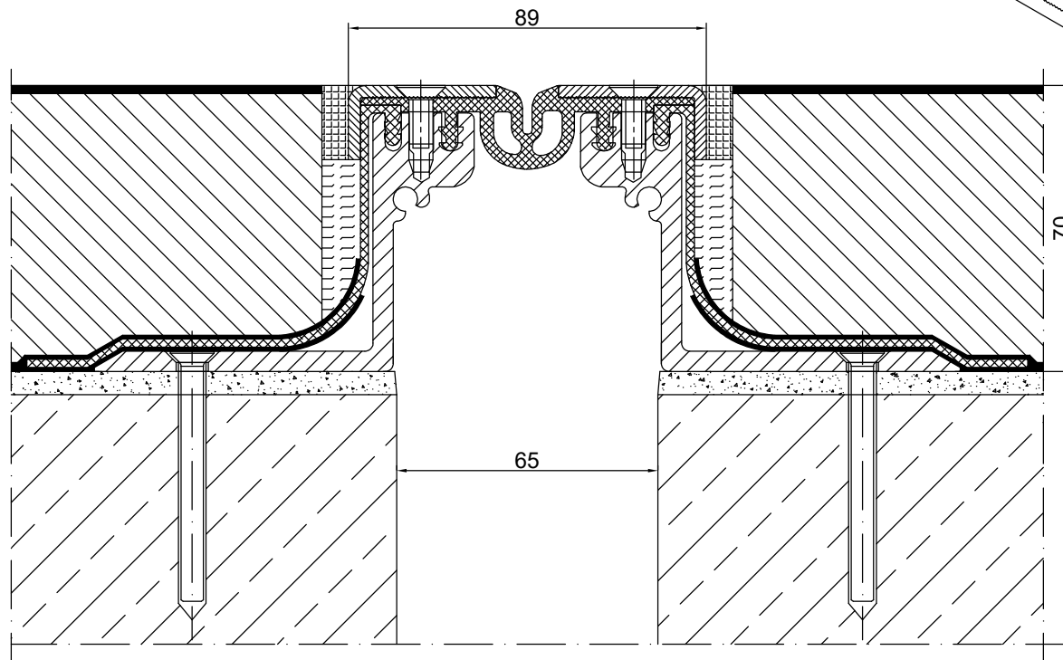
CONECTO GA 43.10.70 L SECTION
