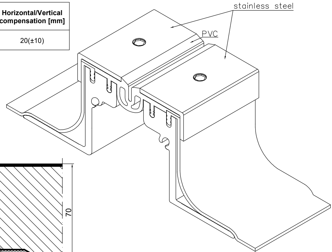
CONECTO GA 43.10.70 L VIEW
