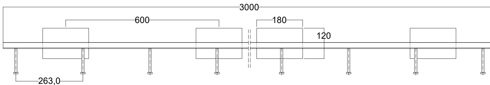
Conecto Omega 03NB-5D-T8 h=175/190 Top view skala 1:1,25
