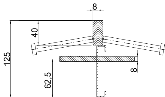
CONECTO DOWEL 08NA40-5D-T8 h=125 SECTION
